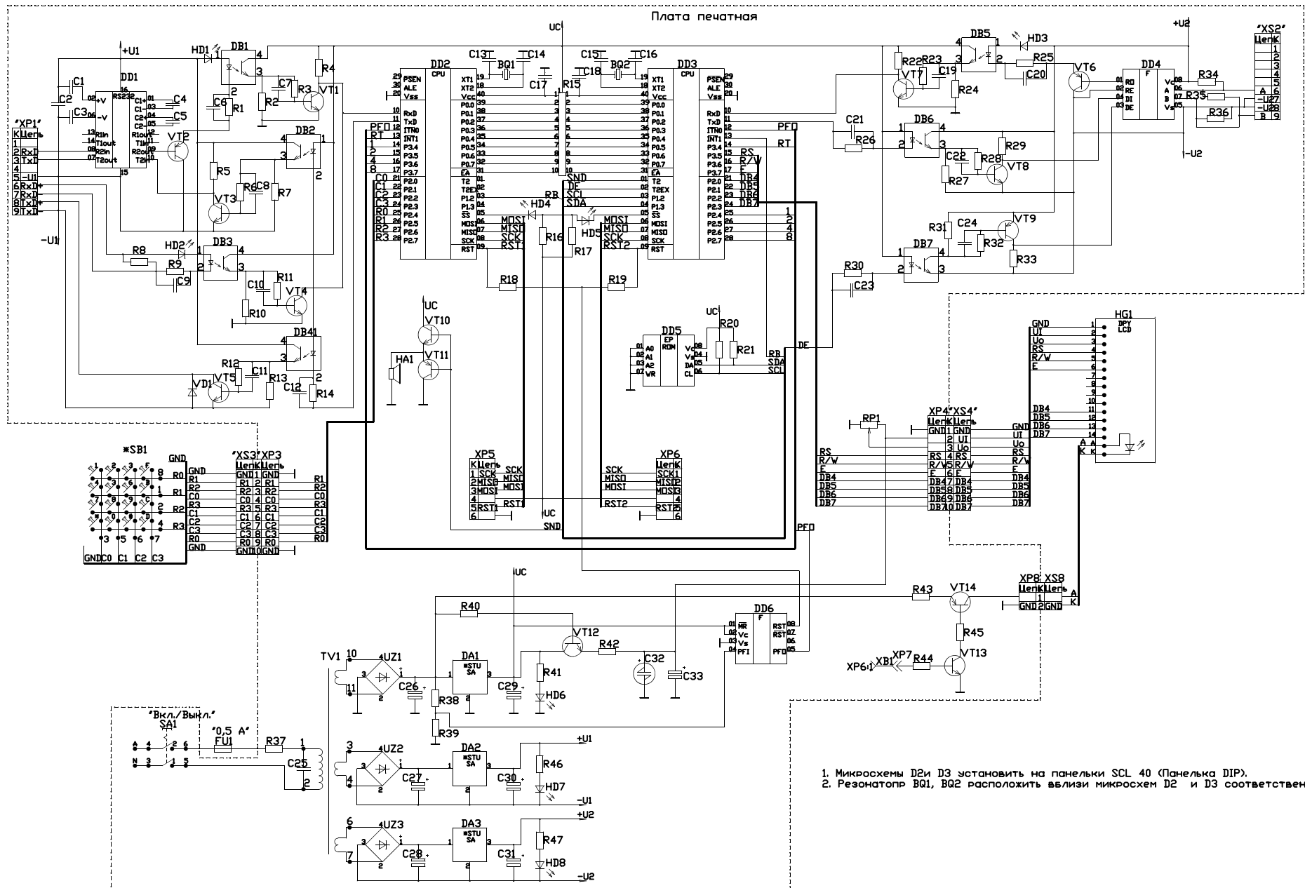
Схема электрическая принципиальная контроллера управления ТРК Агат-12 мк4
