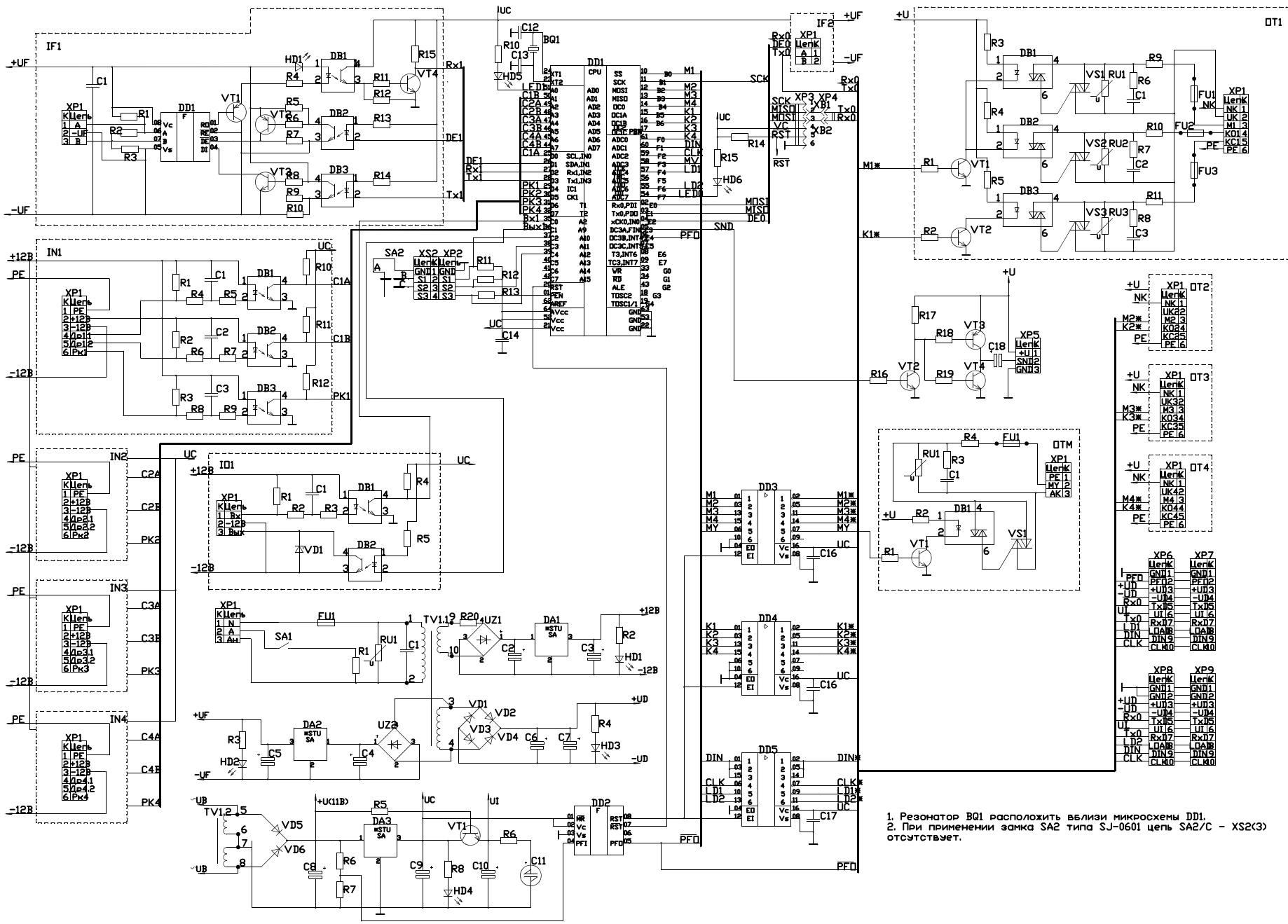
Схема электрическая принципиальная платы управления Агат-4К
